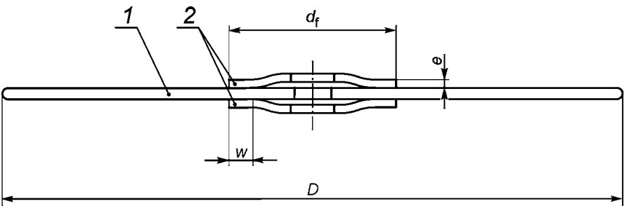
1 — отрезной диск; 2 — фланцы
