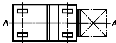
А-А — продольная вертикальная плоскость погрузчика
