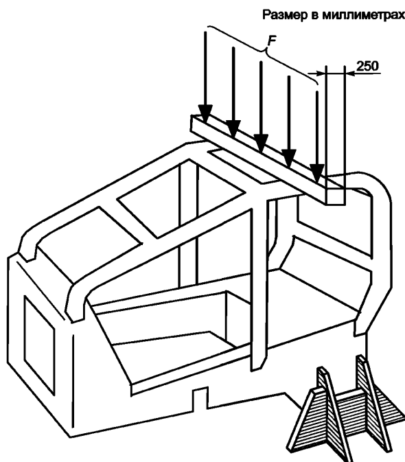
Рисунок 7 — Вертикальное нагружение
