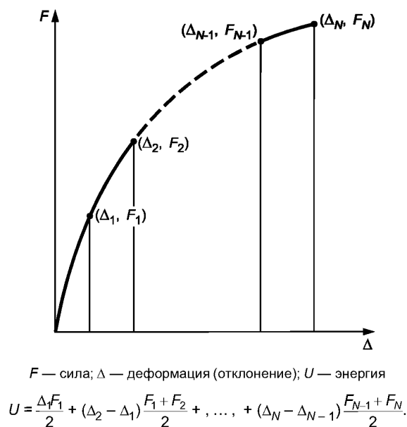
Рисунок 6 — График «деформация — усилие» при боковом нагружении
