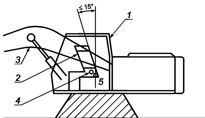
1 — ROPS; 2 — DLV; 3 — жесткие части машины; 4 — SIP; 5 — LA
