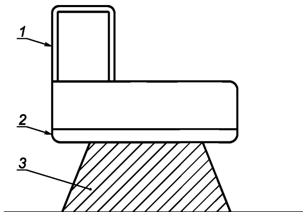
1 — ROPS; 2 — вращающаяся платформа; 3 — опорная плита
