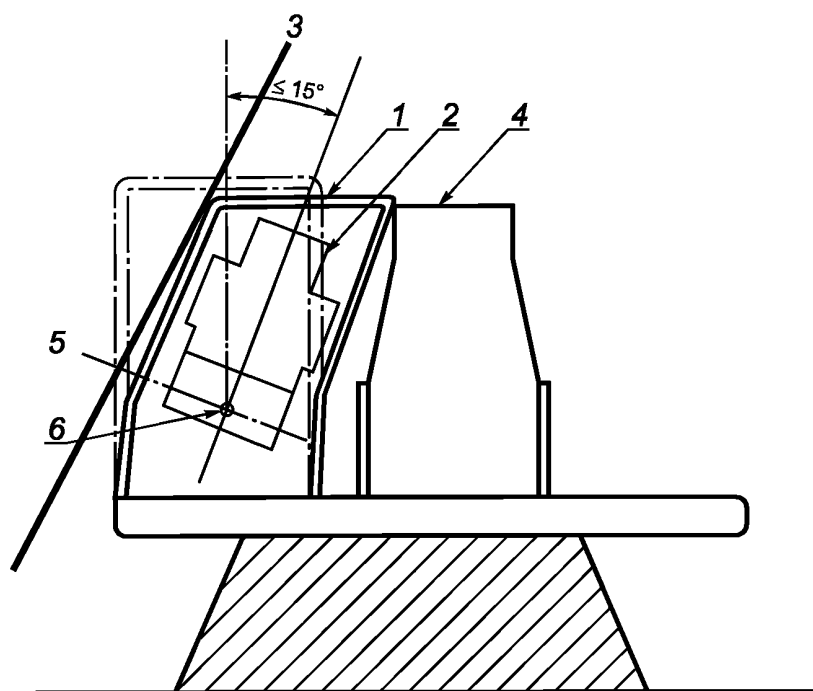
1 — ROPS; 2 — DLV; 3 — LS GP; 4 — жесткие части машины; 5 — LA; 6 — SIP
