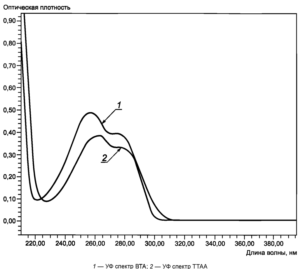
Рисунок В.1 — УФ спектры ТТАА и ВТА
