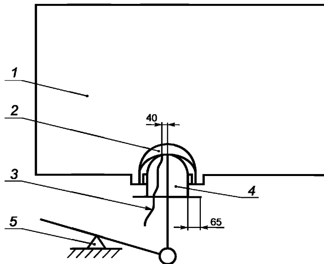
1 — термокамера; 2 — испытываемый образец; 3 — термопара; 4 — термомакет; 5 — подъемное устройство
