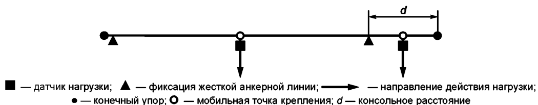
Рисунок 17 — Пример организации испытаний анкерного устройства типа D с консольной балкой
