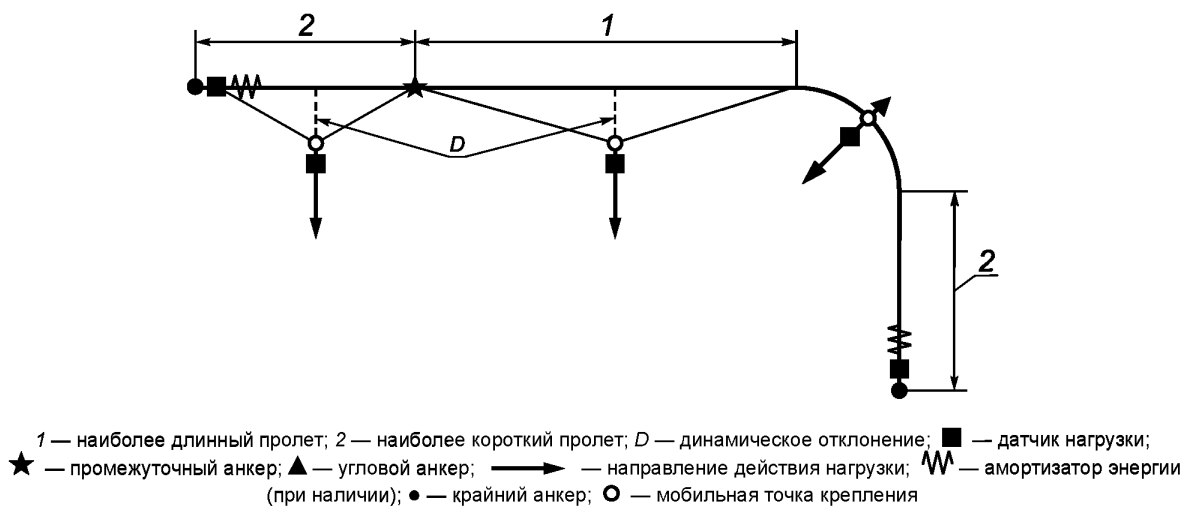
Рисунок 16 — Пример организации испытаний многопролетного анкерного устройства типа С с угловым анкером
