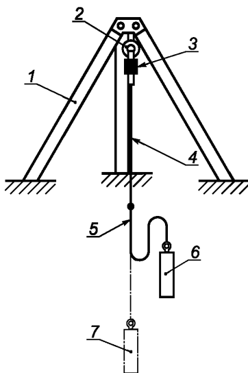
1 — тренога; 2 — точка(и) крепления не на ноге; 3 — датчик нагрузки; 4 — соединительная линия; 5 — строп для испытаний; 6 — положение испытательного груза перед отпусанием; 7 — положение испытательного груза после отпусания
