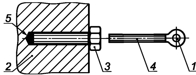
Рисунок 4 — Пример анкерного устройства типа А со структурным анкером
