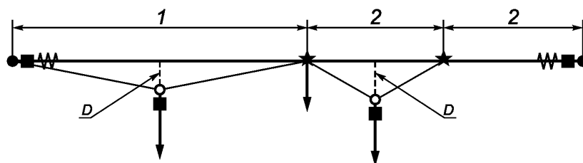
1 — наиболее длинный пролет; 2 — наиболее короткий пролет; D — динамическое отклонение; ■ — датчик нагрузки; ★ — промежуточный анкер; ○ — мобильная точка крепления; —> — направление действия нагрузки; M — амортизатор энергии (при наличии); ● — крайний анкер
