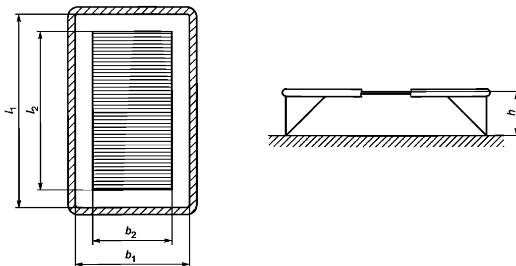
Рисунок 1 — Размеры батуты класса 1
