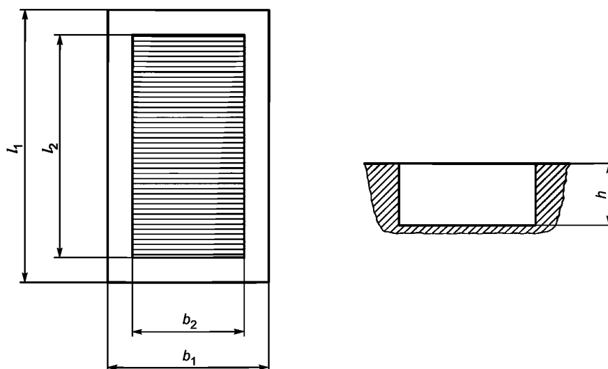
Рисунок 5 — Размеры батутов класса 5
