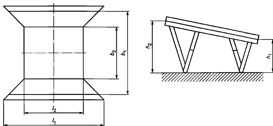
Рисунок 3 — Размеры батуты класса 3
