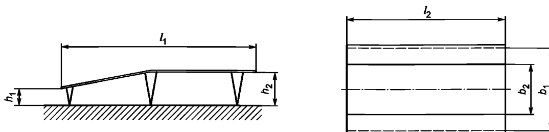
Рисунок 4 — Размеры батутов класса 4
