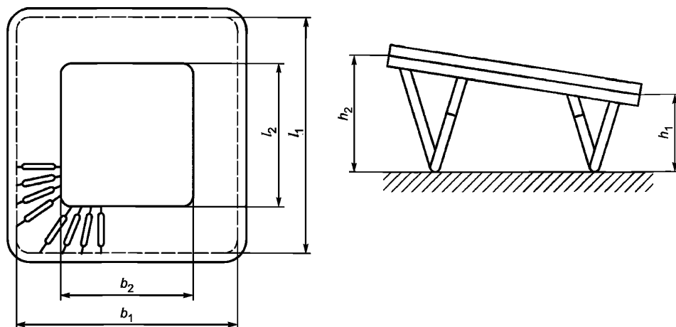
Рисунок 2 — Размеры батуты класса 2
