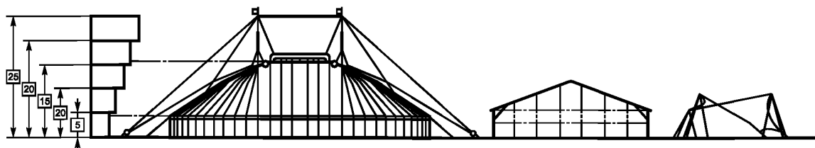
Рисунок 1 — Распределение ветровых нагрузок
