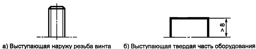
Рисунок 3 — Примеры недопустимых выступающих элементов оборудования
