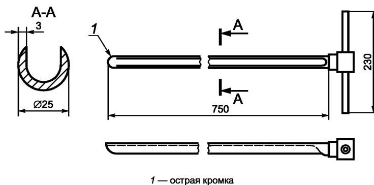
Рисунок 2 — Пробоотборник открытого типа — типичные размеры
