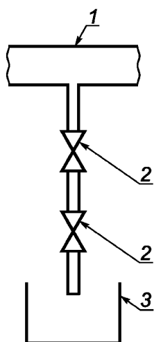
Рисунок 10 — Пробоотборник в виде трубопровода с двойным краном
