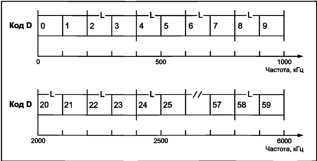
Рисунок 2 — Распределение каналов и рекомендуемые несущие L при использовании полосы аудиочастот в соответствии с таблицей 1
