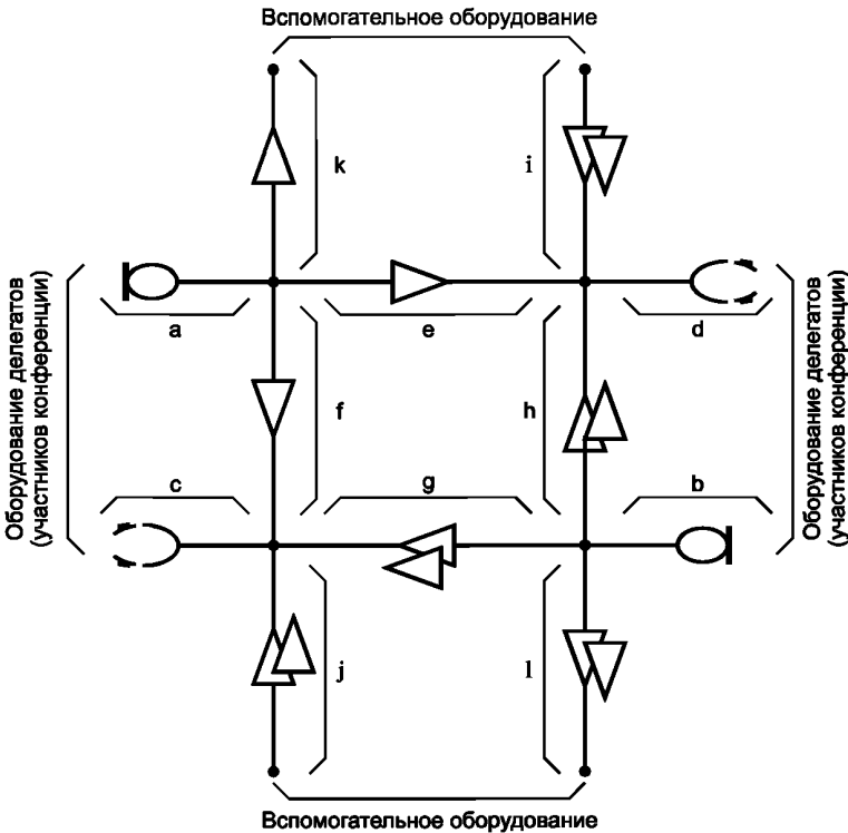
Рисунок 1 — Схемное представление звуковой системы конференц-связи
