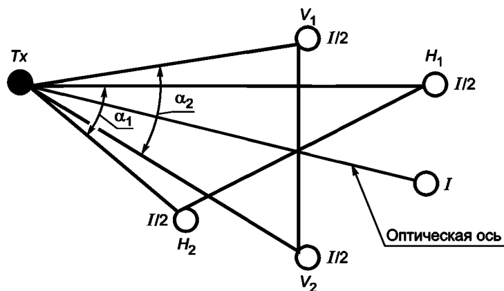
Рисунок 4 — Угол максимальной дивергенции при половине силы оптического излучения
