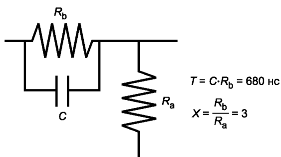
Рисунок 14 — Схема предсказания (пример)
