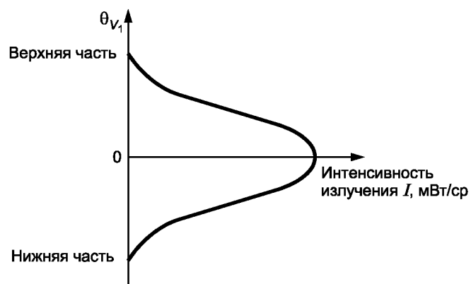
8b — Направленность по вертикали
