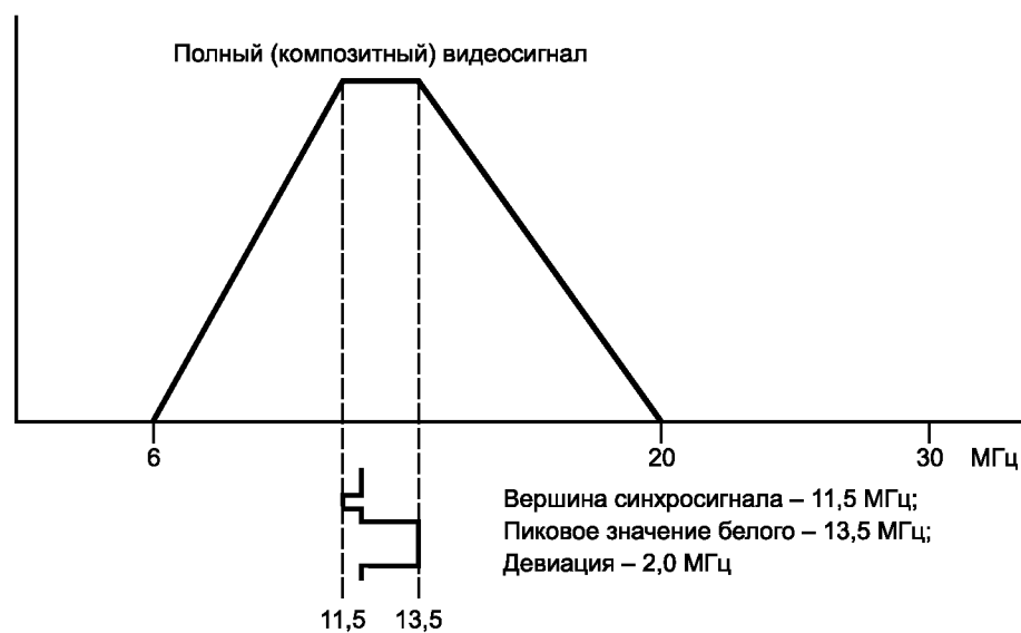
Рисунок 12 — Формат передачи [полный (композитный) видеосигнал]
