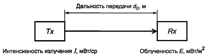
Рисунок 2 — Размещение при измерении
