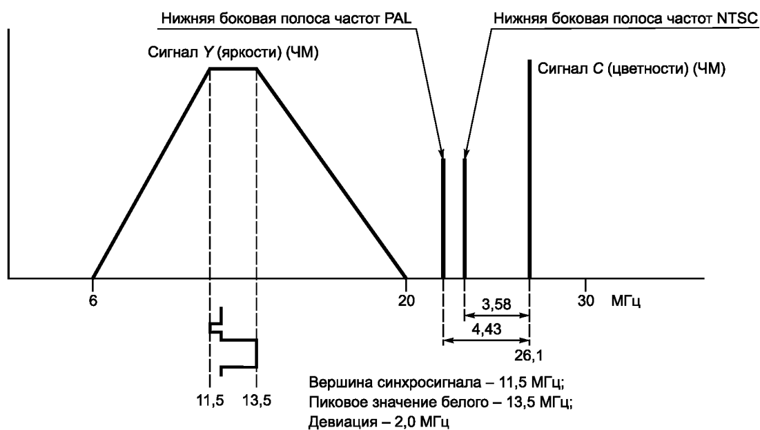
Рисунок 13 — Формат передачи (видеосигнал Y/C с разделением)
