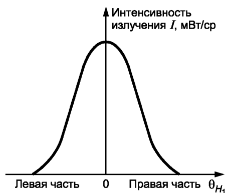
8a — Направленность по горизонтали
