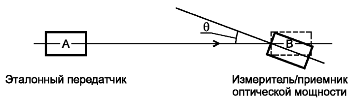
Рисунок 9 — Характеристики приемника
