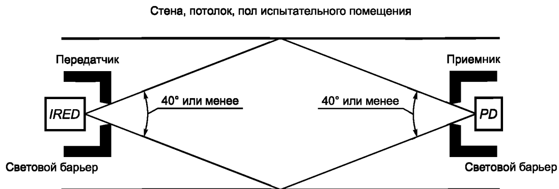
Рисунок 2 — Размещение при измерении
