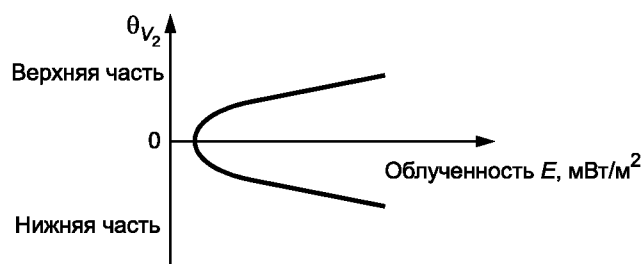
10b — Направленность по вертикали
