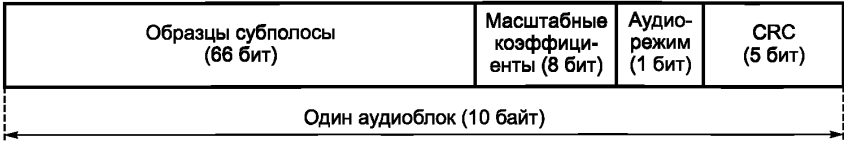
Рисунок 11 — Структура аудиоблока
