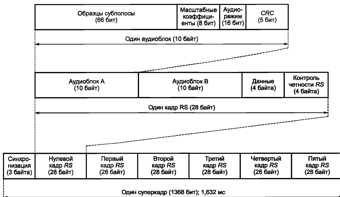
Рисунок 9 — Структура суперкадра
