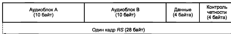
Рисунок 10 — Структура RS-кадра
