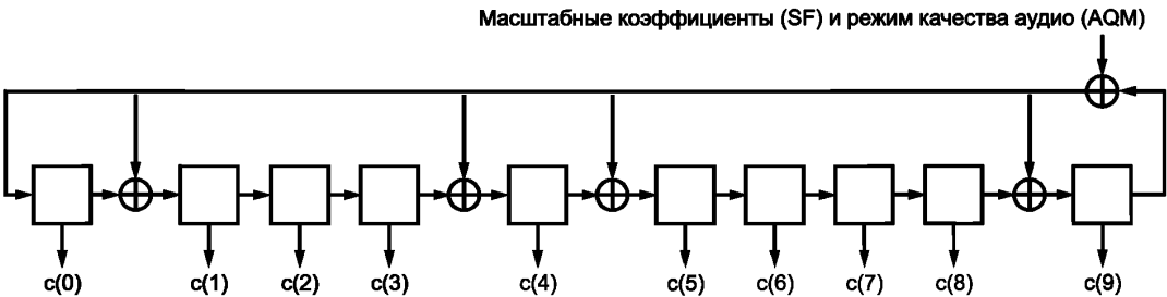
Рисунок 12 — Расчет CRC
