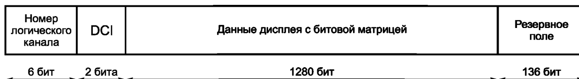
Рисунок 21 — Структура сообщения дисплею при данных дисплею с битовой матрицей
