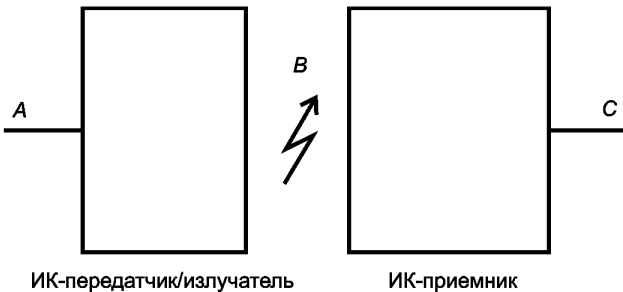
Рисунок 22 — Канал передачи
