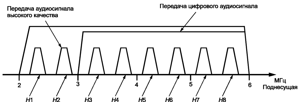
Рисунок 3 — Распределение полосы
