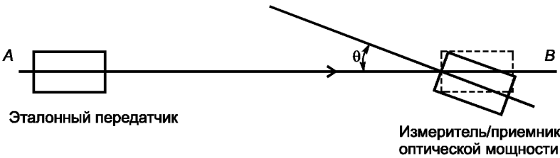
Рисунок 30 — Характеристики приемника
