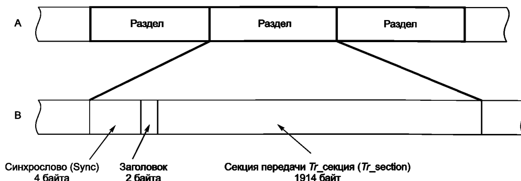
Рисунок 14 — Поток передачи
