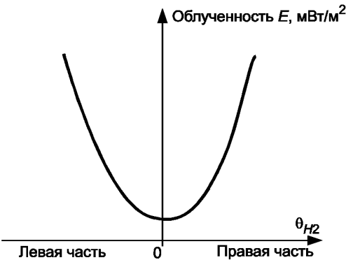
Рисунок 31a — Направленность по горизонтали
