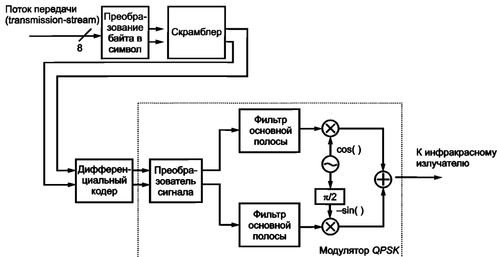
Рисунок 16 — Блок модуляции
