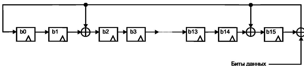
Рисунок В.3 — Схема регистра сдвига с линейной обратной связью
