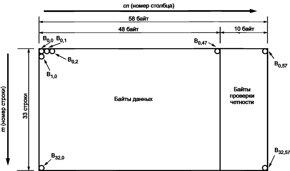
Рисунок 7 — Структура блока
