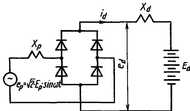
Рассматриваемая схема выпрямителя
