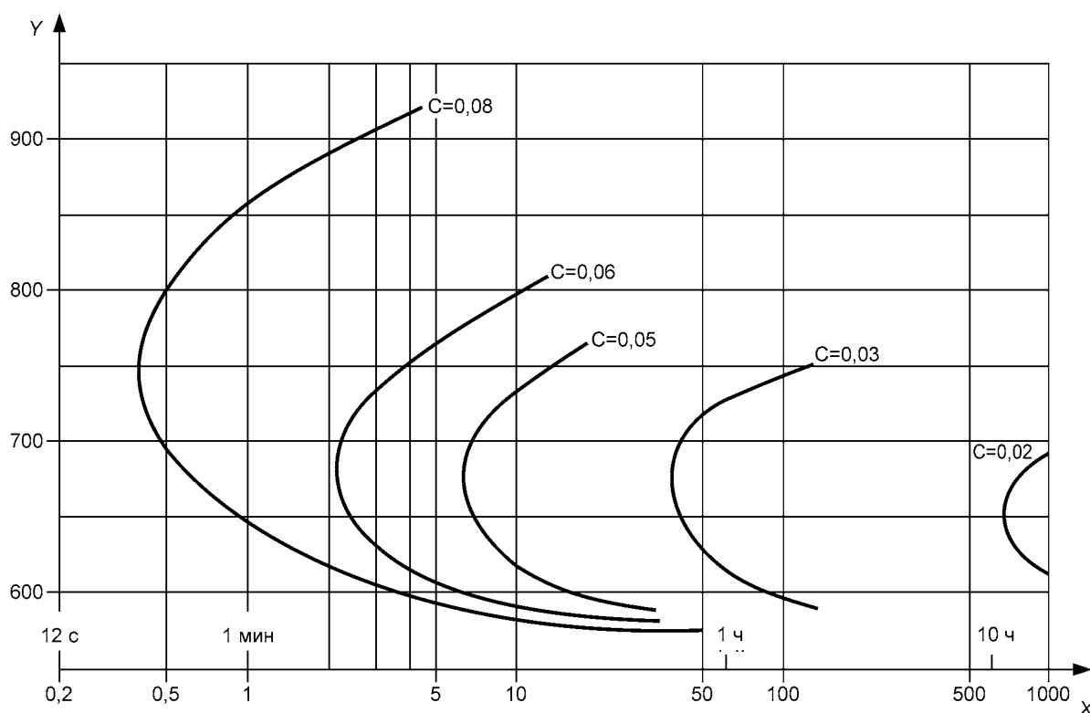
Рисунок F.1 — Температурно-временная диаграмма межкристаллитной коррозии в аустенитной нержавеющей стали марки А2
