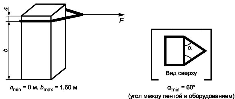
Рисунок 4 — Схема для испытания на устойчивость
