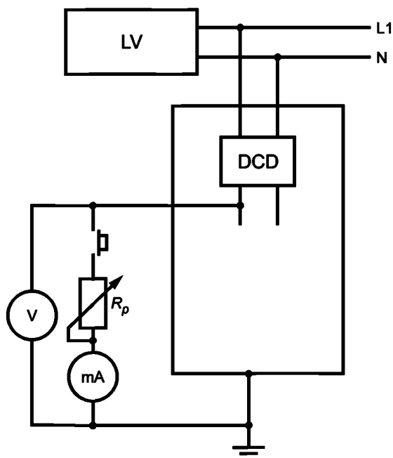
Рисунок 2 — Проверка работы устройства защитного отключения, управляемого дифференциальным током
