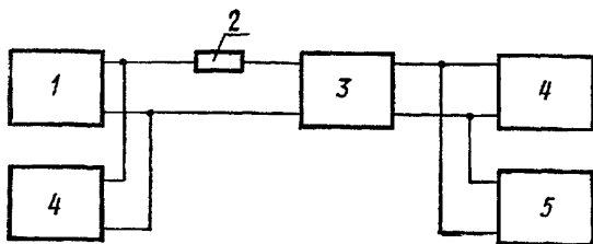
Определение амплитудной и амплитудно-частотной характеристики согласующего усилителя:
