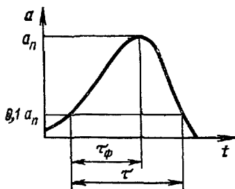
Форма кривой ударного ускорения, воспроизводимого ударной установкой
