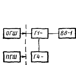
Рис. 1. Структурная схема установки для поверки ГШ с использованием приборов вида Г1: ОГШ — образцовый ГШ; ПГШ — проверяемый ГШ
