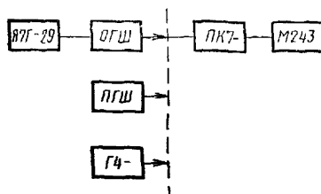
Рис. 2. Структурная схема установки для поверки ГШ с использованием измерителей вида ПК7
