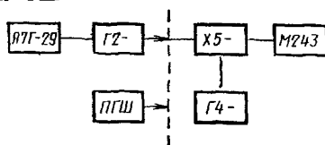
Рис. 3. Структурная схема установки для поверки ГШ с использованием измерителей коэффициента шума
