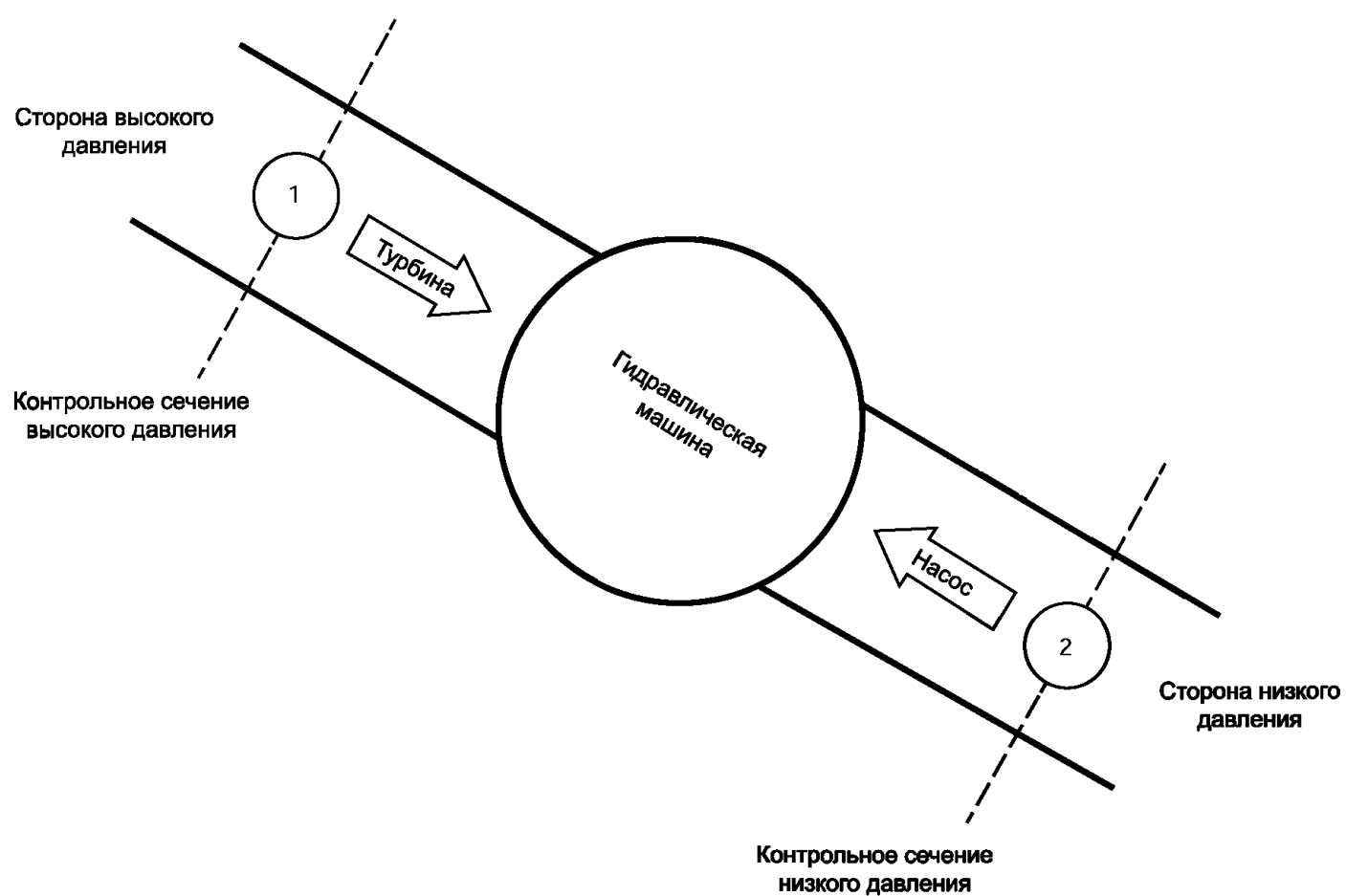
Рисунок 2 — Схематичное представление гидравлической машины
