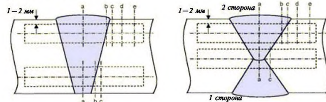
Рис. 6.4.4.4-3 Схема вырезки и расположения надреза на образцах для испытаний на ударный изгиб для технологических процессов сварки с погонной энергией > 50 кДж/см:
