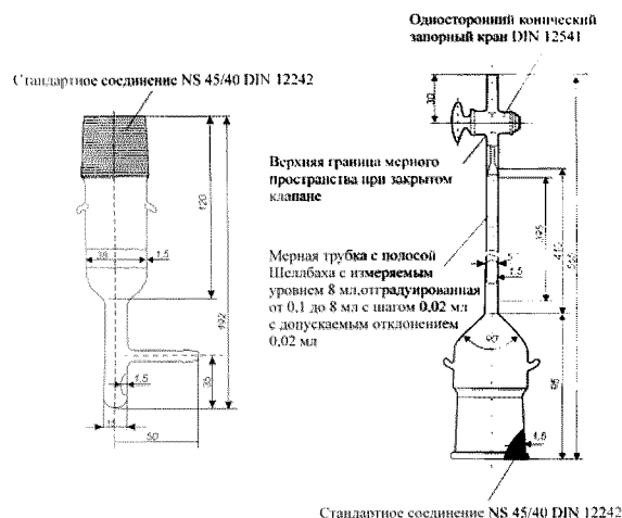
Рис. 5.4.6.6.1-2 Газовая бюретка для определения содержания диффузионного водорода
