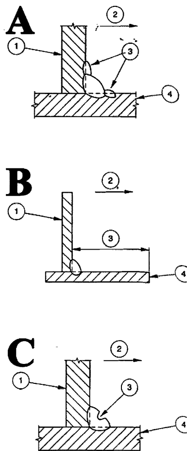
Рис. 5.4.5.3-2 Альтернативные методы локализации мест разрушения углового шва.
