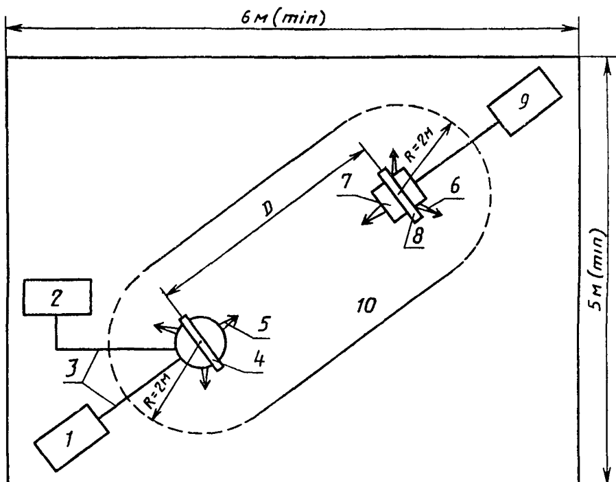
Рис. 1. Рекомендуемое размещение аппаратуры при поверке ИМП:
