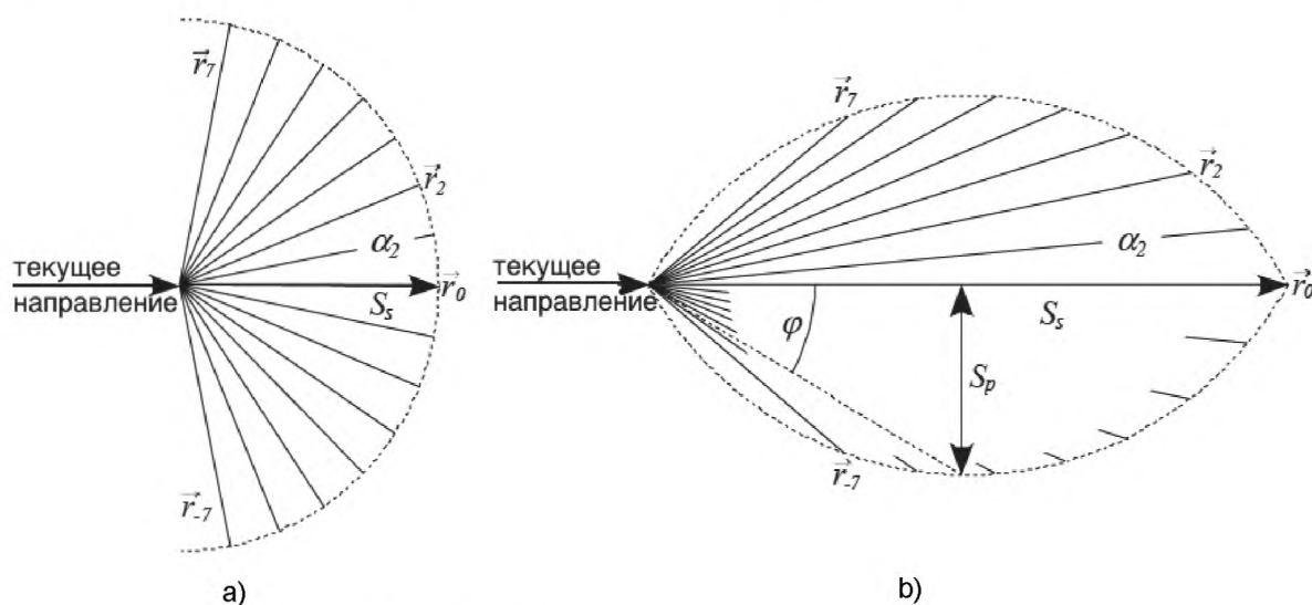
Рисунок 5 — Длина шага, зависящая от направления:
