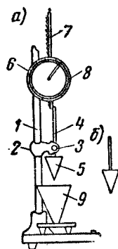
Рис. 1. Прибор для определения подвижности раствора
