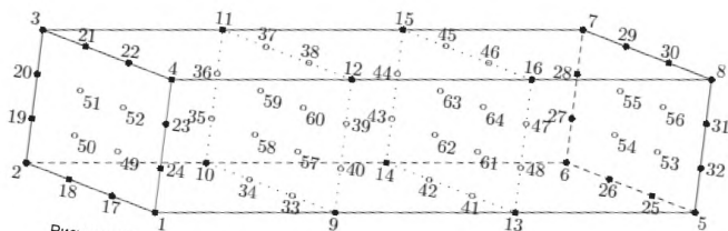
Рисунок 17 — Линейные, квадратичные и кубические шестигранные ячейки
