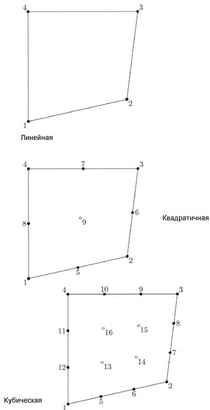
Рисунок 16 — Линейные, квадратичные и кубические четырехугольные ячейки
