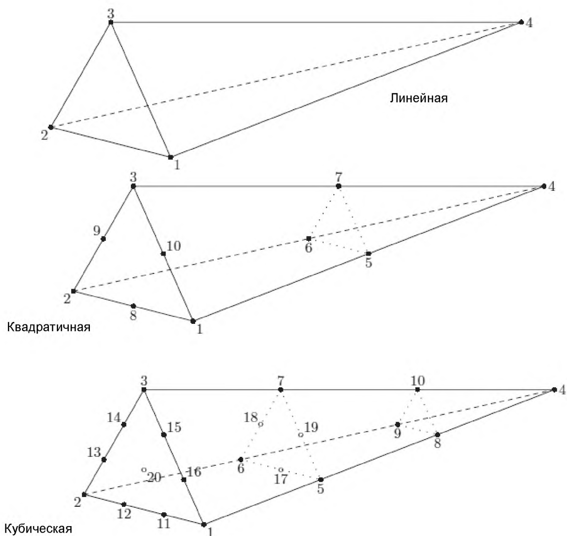
Рисунок 19 — Линейные, квадратичные и кубические тетраэдральные ячейки
