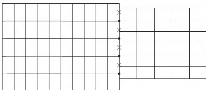
Рисунок 22 — Рассогласованный граничащий стык
