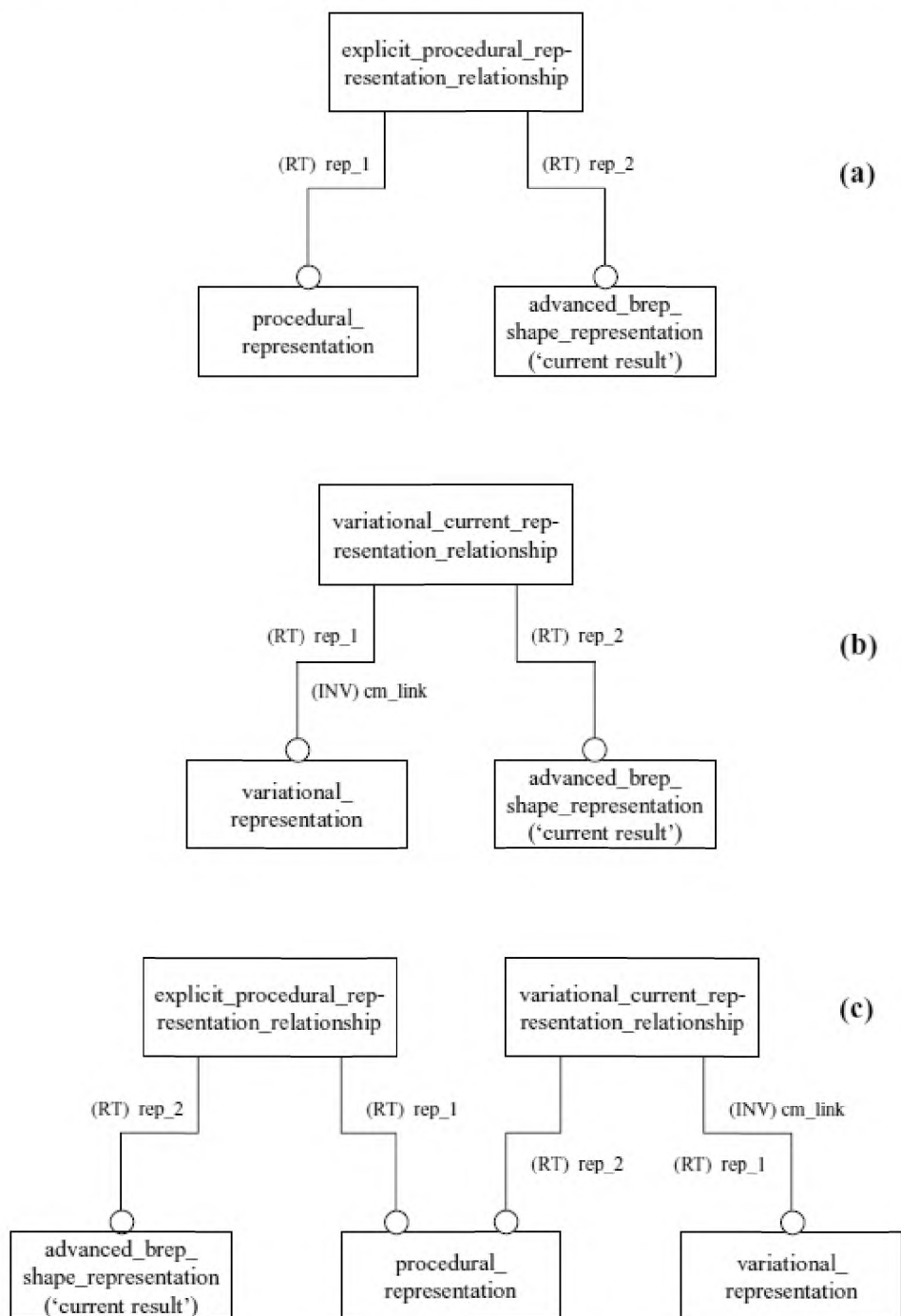
Рисунок Е.1 – Взаимосвязи между экземплярами процедурной, вариационной и явно заданной моделей для комбинаций (а) – без вариационной модели, (b) – без процедурной модели и (с) – наличие всех трех моделей
