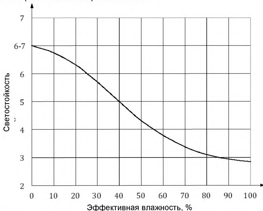
Рисунок 1 — Средние значения, полученные при экспонировании для контроля влажности
