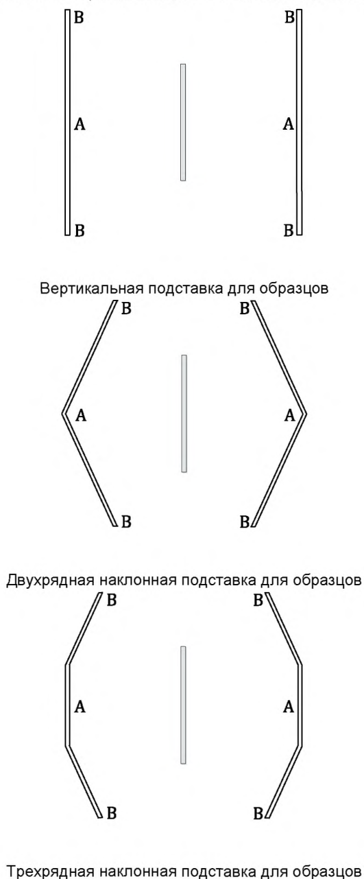
Рисунок В.1 — Определение равномерности энергетической освещенности в устройствах для экспонирования, использующих вращающуюся подставку для образцов
