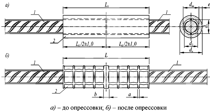
Рисунок 1 – Растянутое стандартное соединение стержневой арматуры
