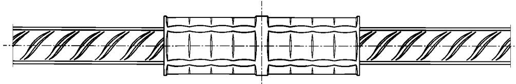
Рисунок А.2 – Растянутое соединение, опрессованное без промежутков
