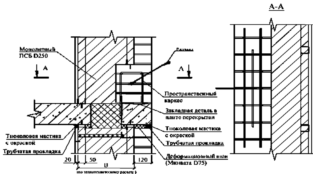
Устройство для крепления кронштейна
