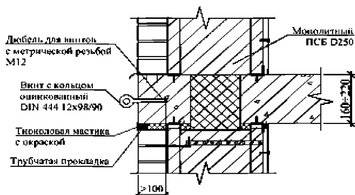
Устройство для крепления растяжек (при расчетном обосновании)
