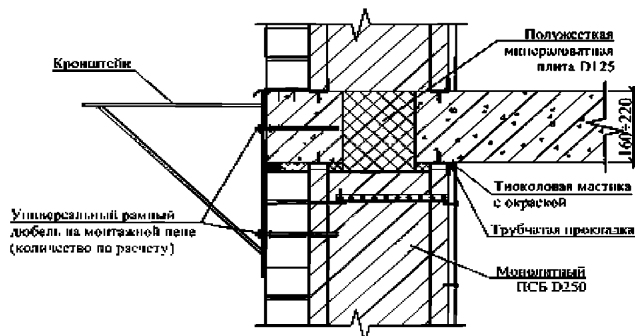
Устройство для крепления растяжек (при расчетном обосновании)
