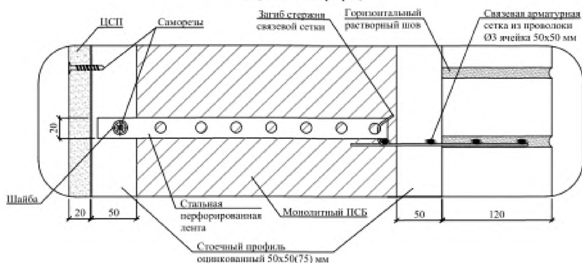
Узел В. Вариант 2 (горизонтальный разрез)
