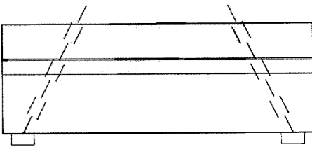
Рисунок 10 – Схема строповки зоны Б
