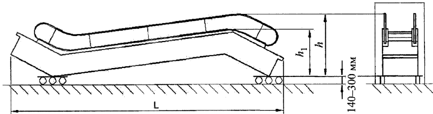
Рисунок 2 – Габаритные размеры эскалатора в сборе
