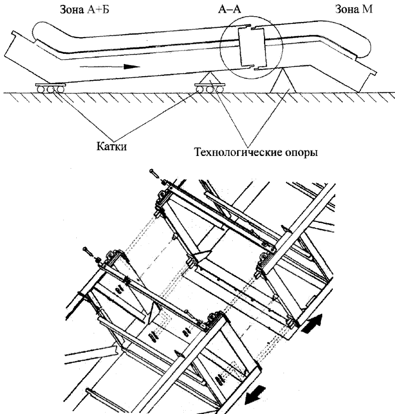
Рисунок 14 – Схема соединения зон М и А+Б
