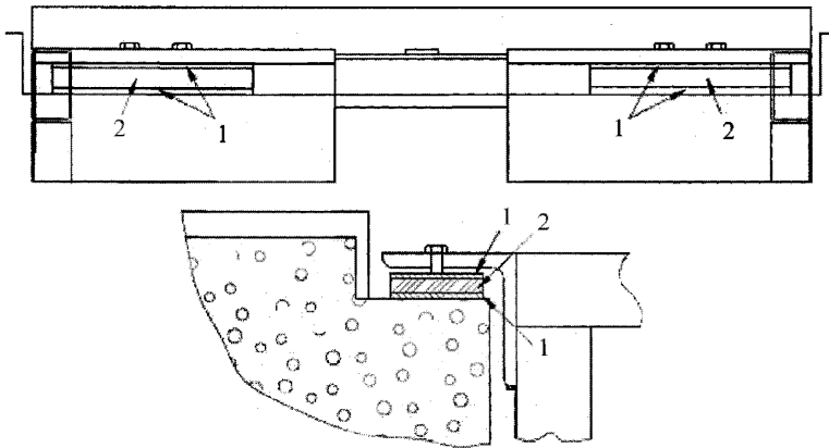
1 – опорная пластина; 2 – резиновый амортизатор
