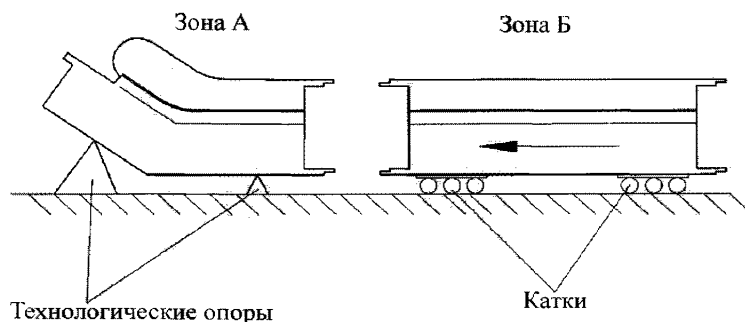
Рисунок 13 – Схема соединения зон А и Б
