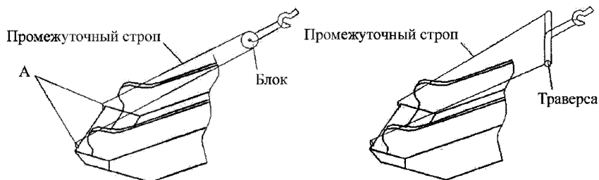
Рисунок 6 – Схемы строповки эскалатора за грузовые скобы
