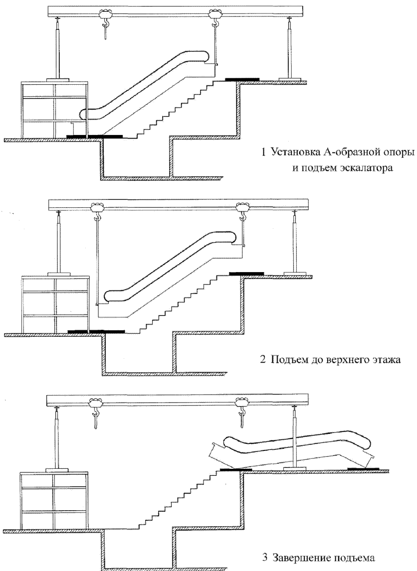
Рисунок 12, лист 2 – Перемещение эскалатора вверх по лестнице с применением А-образной опоры
