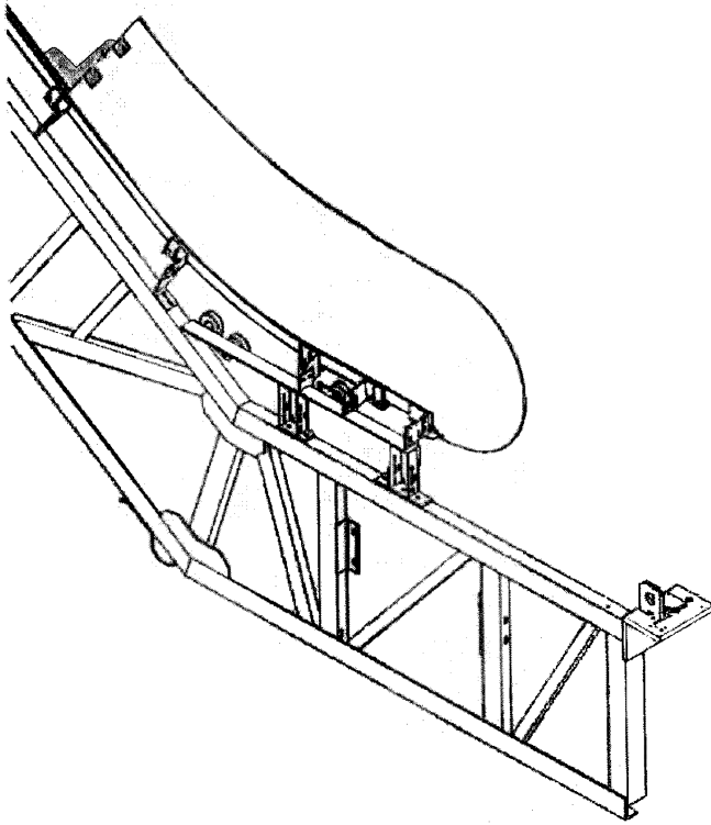
Рисунок 15 – Установка крайней стеклянной панели
