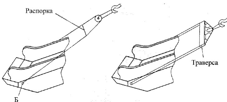
Рисунок 7 – Схемы строповки эскалатора за отверстия в поясах
