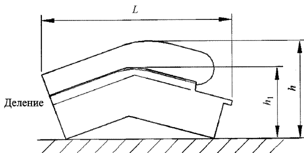
Рисунок 5 – Габаритные размеры зоны М
