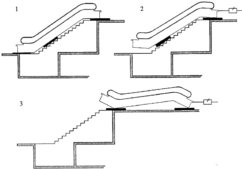
Рисунок 11, лист 2 – Перемещение эскалатора вверх по лестнице с применением настила
