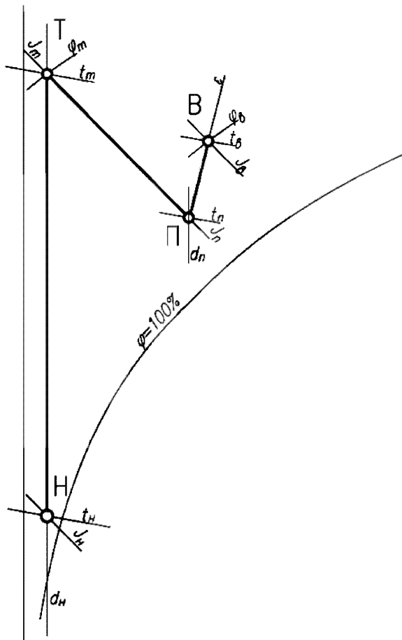
Рисунок 2 – Процесс обработки воздуха в центральных прямооточных СКВ в холодный период года
