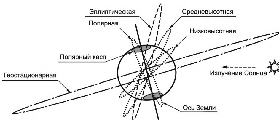
Рисунок В.1 — Типовые орбиты космических аппаратов
