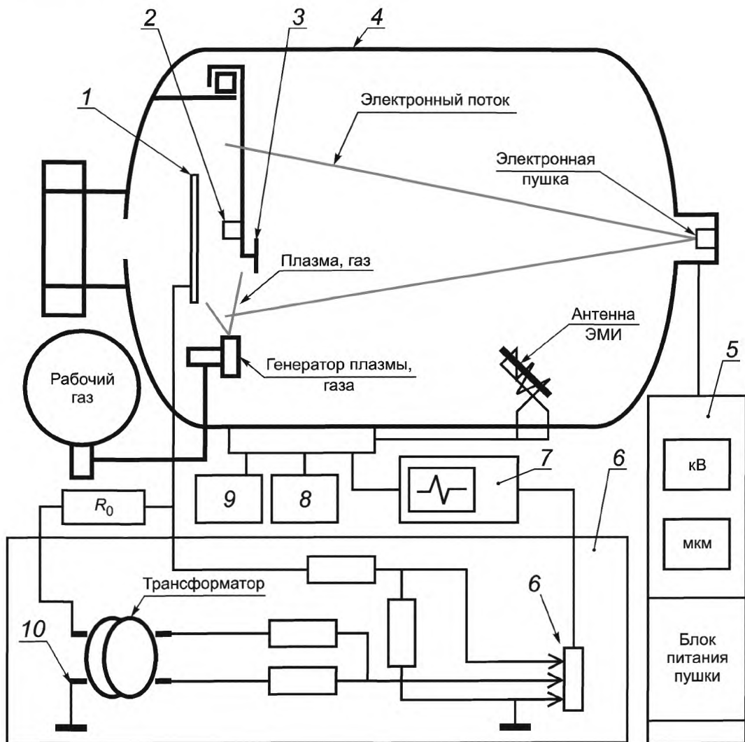
1 — исследуемый образец; 2 — датчик электрического поля на координатном устройстве; 3 — измеритель плотности потока электронов; 4 — вакуумная камера; 5 — блок контроля питания электронной пушки; 6 — электрическая схема измерения импульса тока; 7 — электронно-лучевой запоминающий осциллограф; 8 — осциллограф-регистратор; 9 — ампервольтметр; 10 — цепь заземления, R_0 = 50 \text{ Ом} . ЭМИ — электромагнитный импульс электрического разряда
