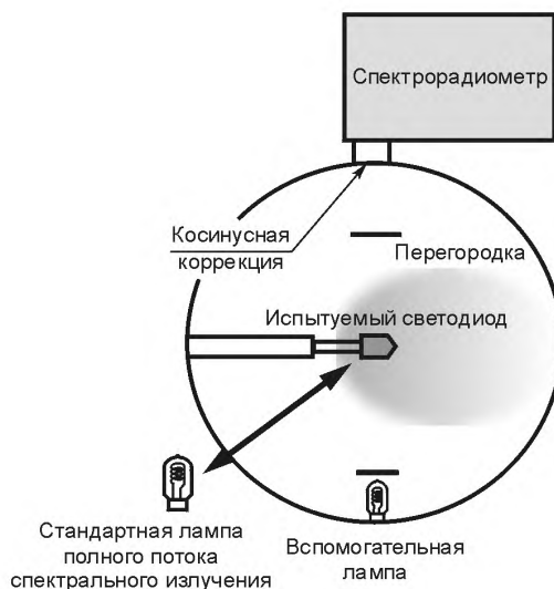
Рисунок 4 — Оптическая схема измерений в режиме полного потока
