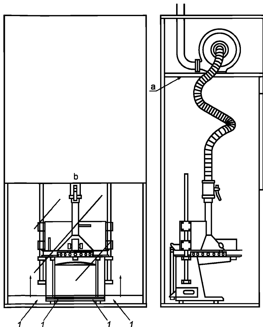
Рисунок А.2 — Шкаф ротационной курительной машины типа а) с колпаком
