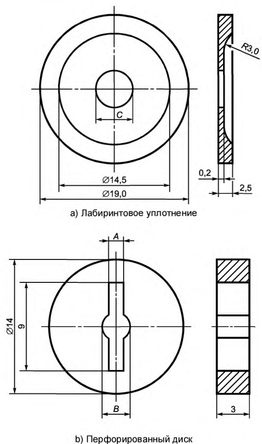
Рисунок 1 — Лабиринтовое уплотнение и перфорированный диск держателя сигарет
