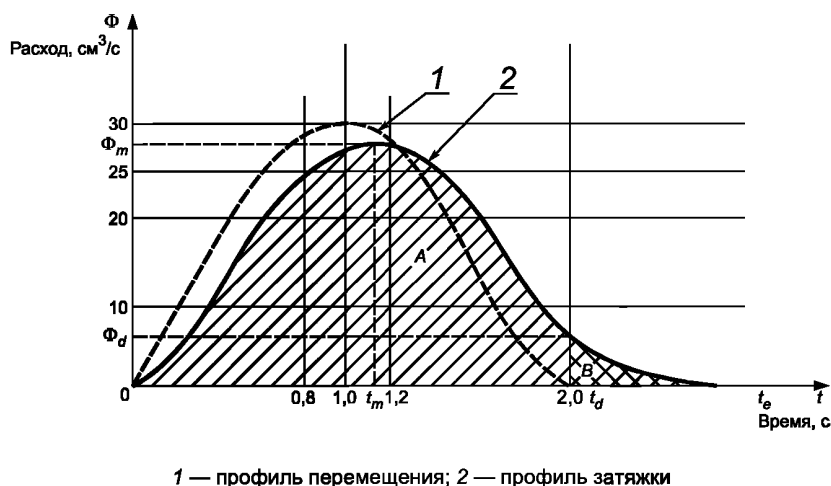
Рисунок С.1 — Схематическое изображение профиля затяжки сигареты
