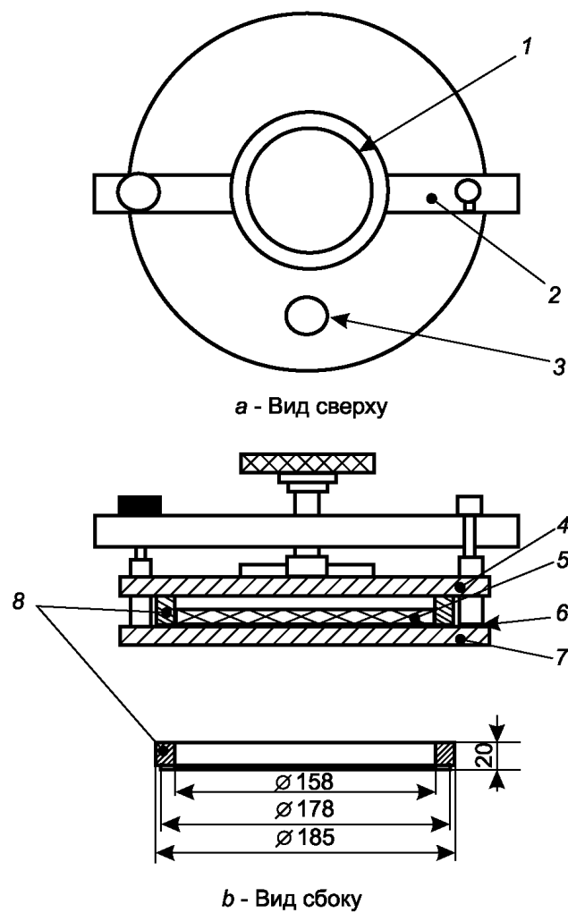
1 – зажимной винт; 2 – прижимная планка; 3 – пробка заливного отверстия; 4 – крышка; 5 – имитатор пищевого продукта; 6 – резиновый коврик; 7 – опорное основание; 8 – уплотнительное кольцо
