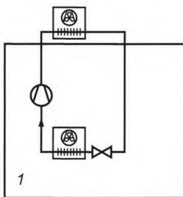
Рисунок С.1 — Холодильная система установлена в том же помещении, что и холодопотребляющий объект
