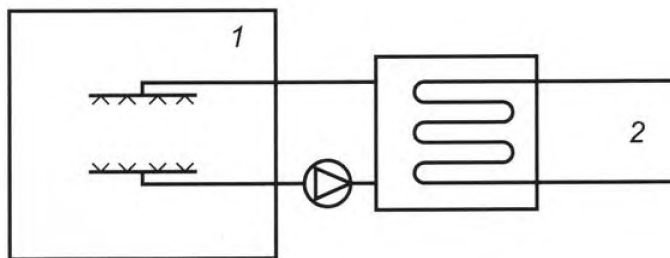
Рисунок 1b — Открытая оросительная система
