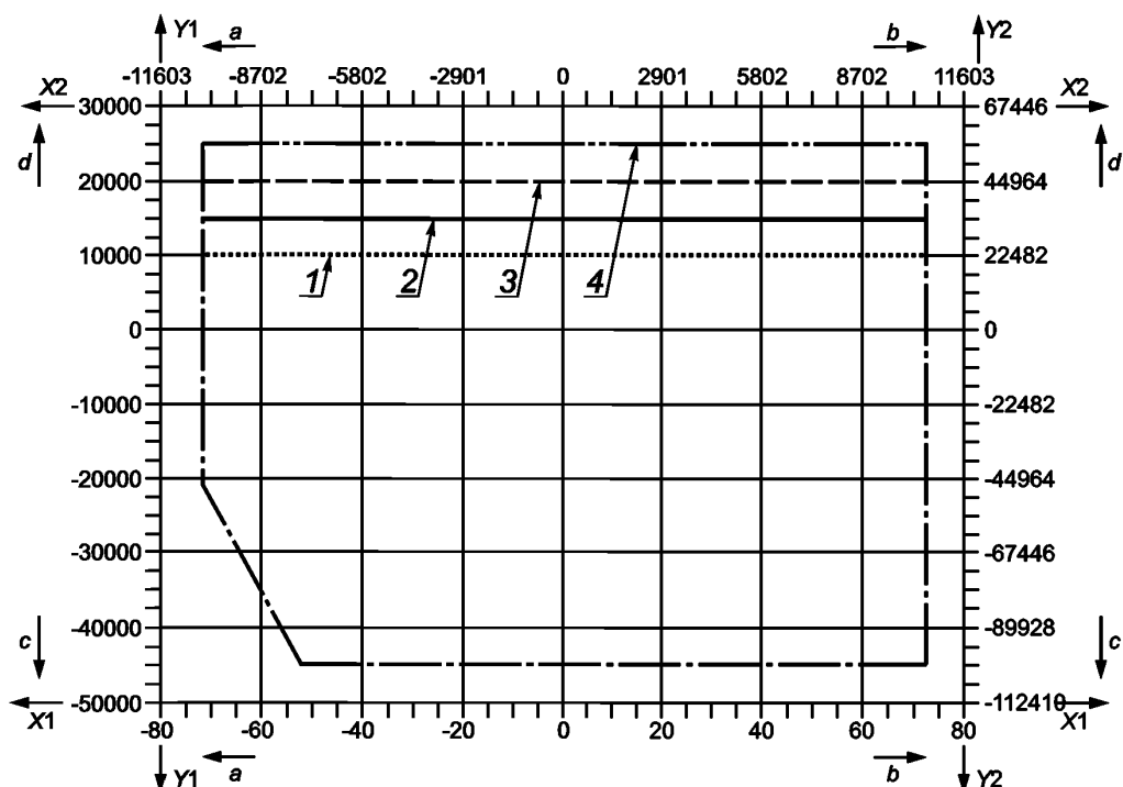
X1 — давление, МПа; X2 — давление, фунт/дюйм 2 ; Y1 — сила, даН; Y2 — сила, фунт; 1 — область для 10 000 даН (212 482 фунт) срез. кольцо; 2 — область для 15 000 даН (33 723 фн) срез. кольцо; 3 — область для 20 000 даН (44 964 фунт) срез. кольцо; 4 — область для 25 000 даН (956 205 фунт) срез. кольца; а — выше; b — ниже; c — сжатие; d — растяжение
