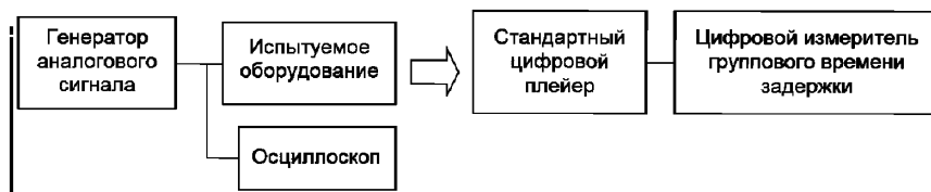
Рисунок 20 — Схема соединения оборудования
