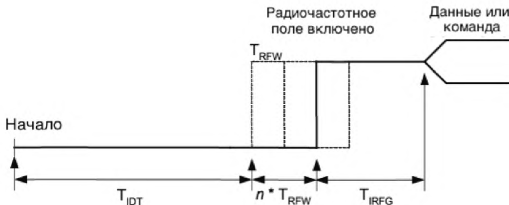
Рисунок 2 — Обнаружение радиочастотного излучения и первоначальная радиочастотная генерация для режима PCD и режима VCD
