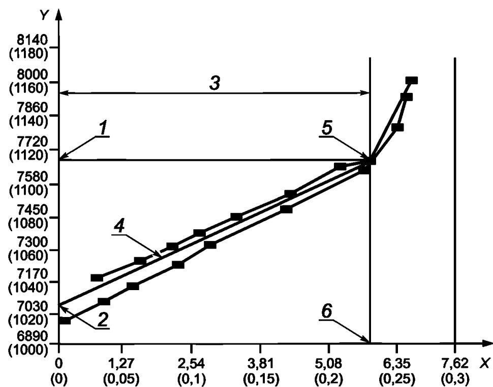
Рисунок G.4 — Пример нанесения данных перемещения штанги
