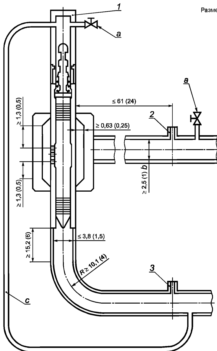
1 — предохранительная головка; 2 — входное давление и датчики температуры; 3 — выходное давление и опционные датчики температуры; а — выпуск в атмосферу перед извлечением клапана (контрольный образец); b — ≤ 61 см (24 дюйма) от контрольного образца; с — уравнильный трубопровод, рекомендованный при применении предохранительной головки
