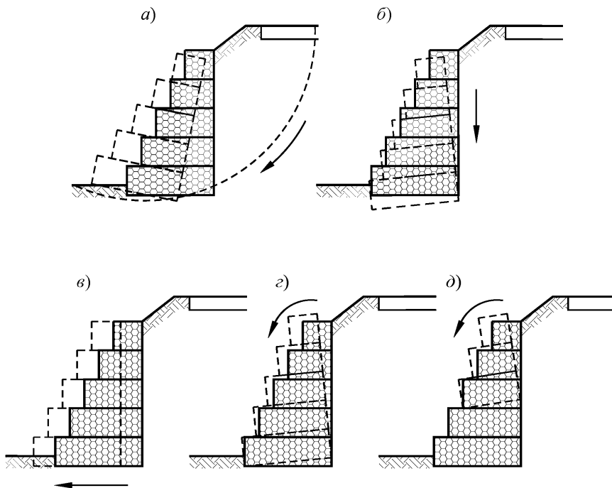
а – нарушение общей устойчивости; б – нарушение несущей способности основания; в – сдвиг; г – опрокидывание; д – внутреннее разрушение
