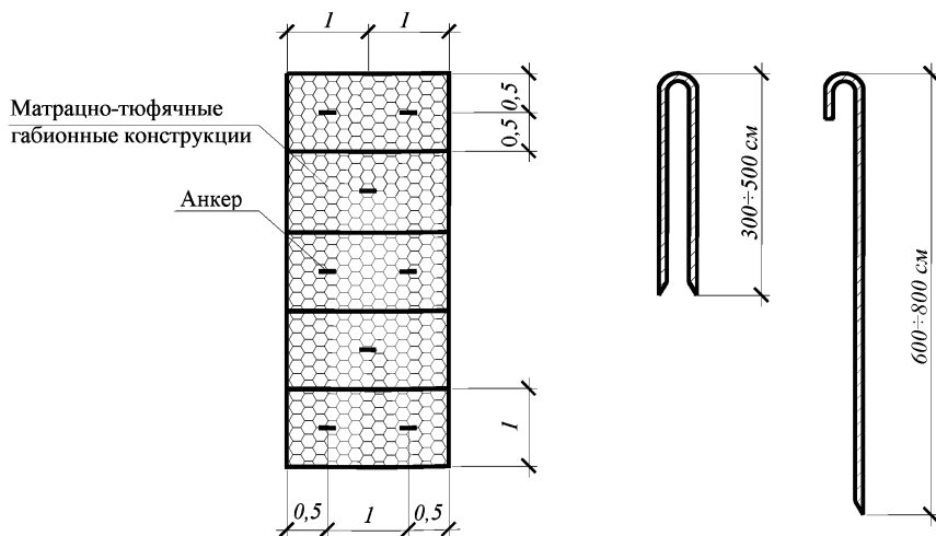
Рисунок 20 – Схема анкеровки матрацно-тюфячной габионной конструкции
