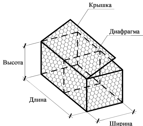
Рисунок 1 – Конструктивная схема габийных конструкций коробчатой формы
