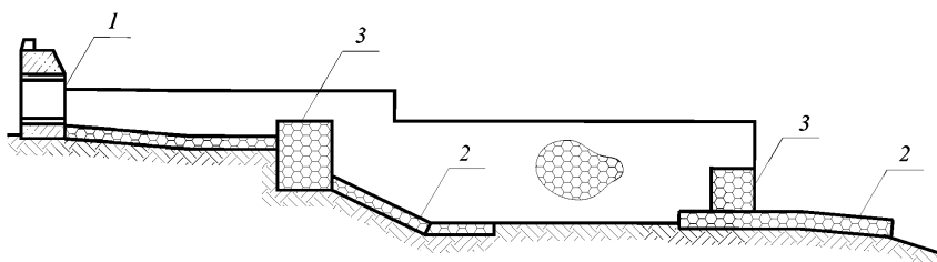
Рисунок 30 – Схемы возможных упорно-защитных габионных устройств в концевых частях входных и выходных русел
