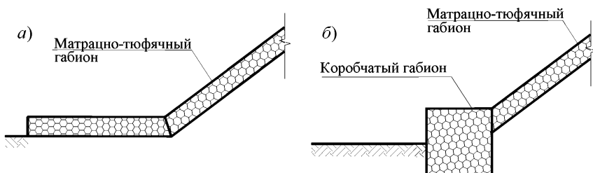
а – упор из матрадно-тюфячного габиона; б – упор из коробчатого габиона
