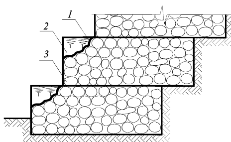
Рисунок 7 – Виды подпорных стен из габионных конструкций
