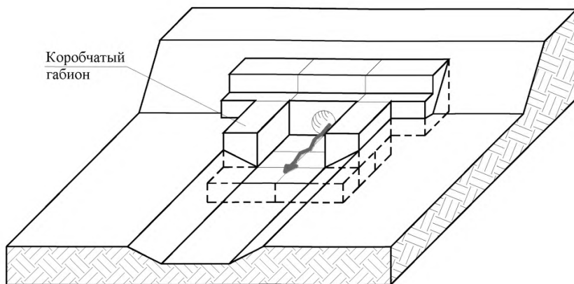
Рисунок 29 – Схемы габионных укреплений выходных оголовков круглых водопропускных труб
