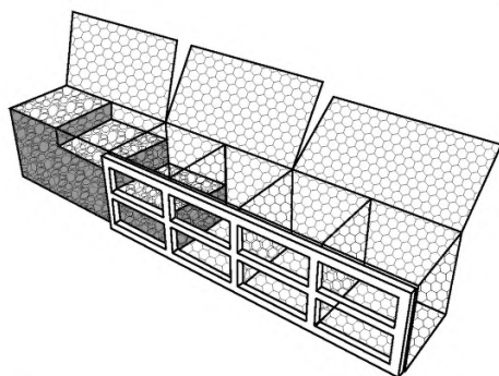
Рисунок 40 – Установка опалубки на коробчатые габионные конструкции
