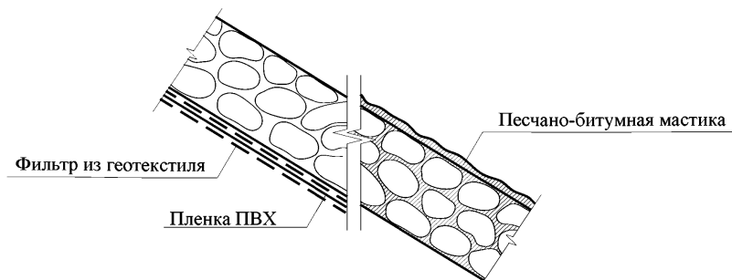
Рисунок 21 – Мероприятия по предотвращению фильтрации дождевых вод через габрионную противозерозионную конструкцию
