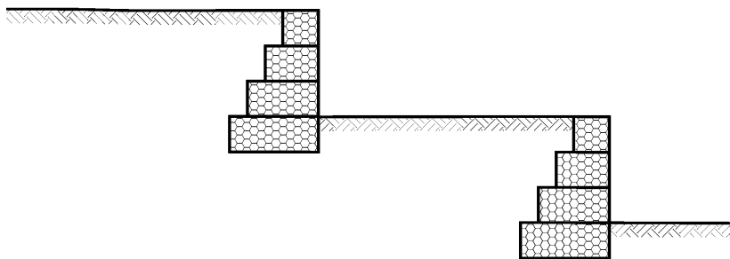
Рисунок 33 – Схемы габионных стабилизирующих противоселевых сооружений
