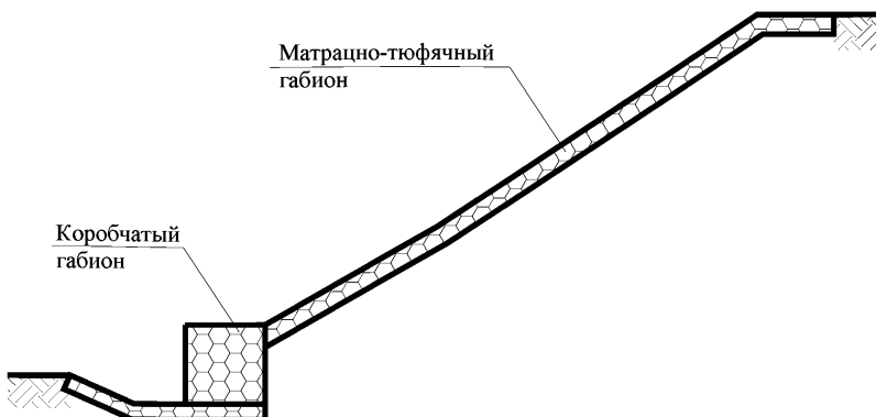
Рисунок 18 – Схема укрепления откоса габионным противозрозионным сооружением
