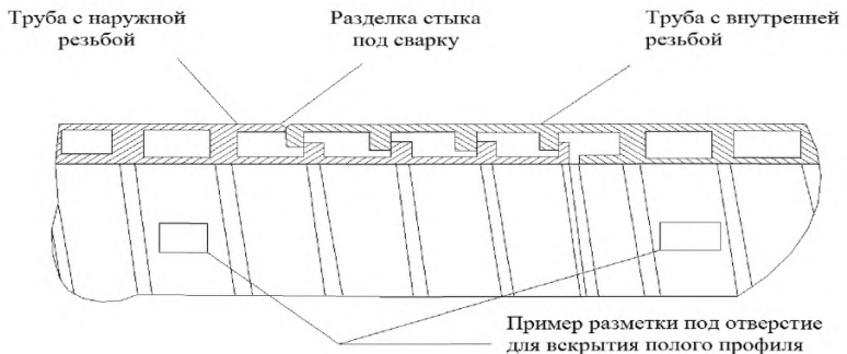
Рисунок 5 – Пример разметки под отверстие для вскрытия полого профиля
