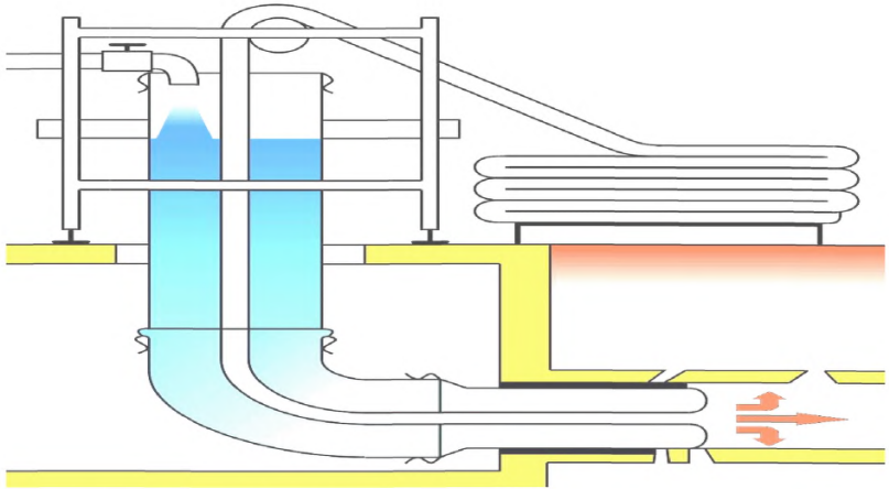
Рисунок 4 – Технология ремонта водопропускной трубы
