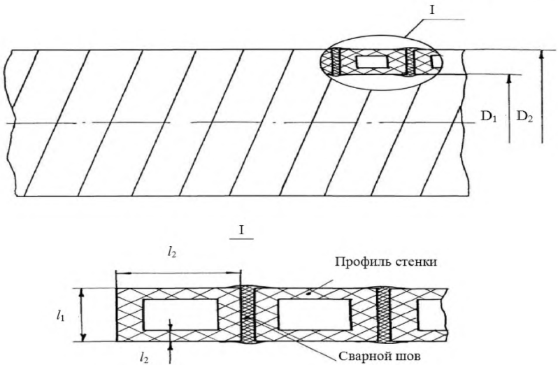
Рисунок 3 – Конструкция спиральновитой трубы из композиционного материала с полой стенкой ( D_1 – внутренний, D_2 – внешний диаметр, h – толщина стенки, l_1 – толщина профиля, l_2 – ширина профиля спиральновитой плиты)
