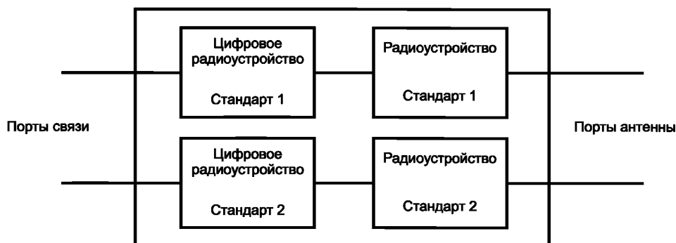
Рисунок 1 — Многокантовое радиооборудование с индивидуальными радиоинтерфейсами
