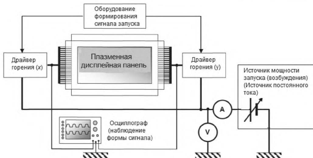
Рисунок 8 – Схема системы измерения мощности запуска (горения)
