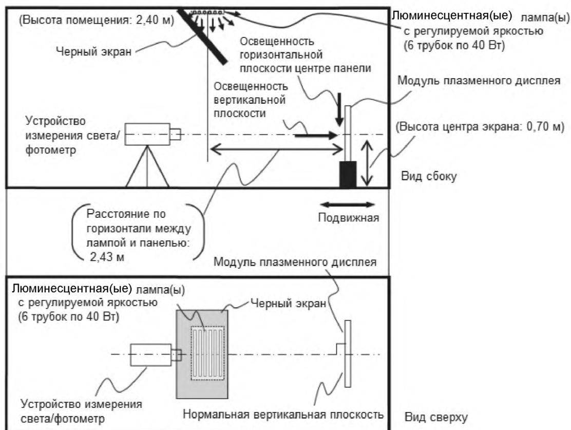
Рисунок 2 — Пример условий освещенного помещения
