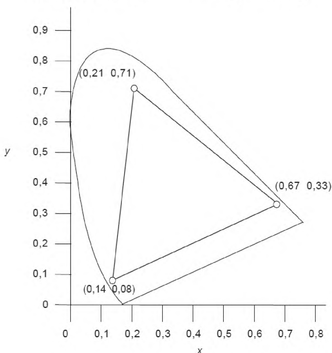
Рисунок 6 – Пример измерения цветовой гаммы
