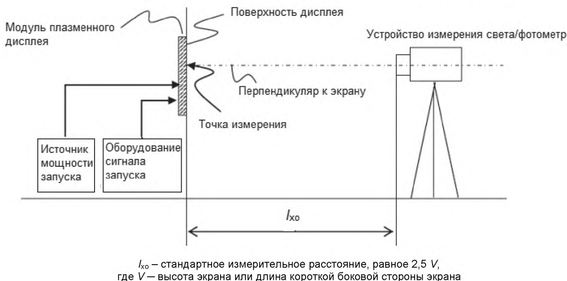
Рисунок 1 — Схема измерения (вид сбоку)
