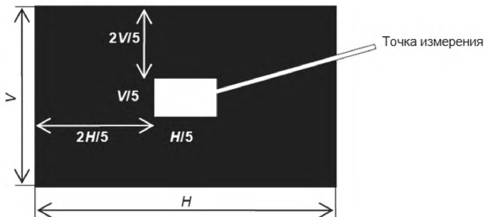
Рисунок 3 – Схема измерения яркости 4 %-ного окна
