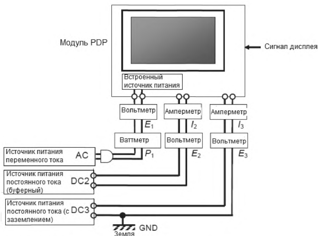
Рисунок 7 – Пример схемы измерения мощности и тока
