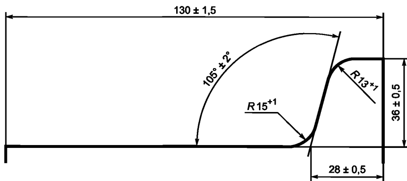
Рисунок 2 — Геометрические размеры профиля обода колеса
