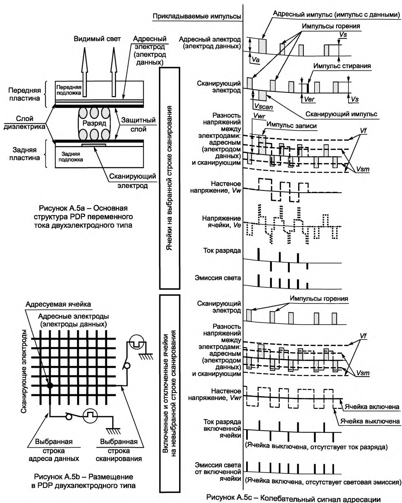
Рисунок А.5 — Работа AC PDP двухэлектродного типа
