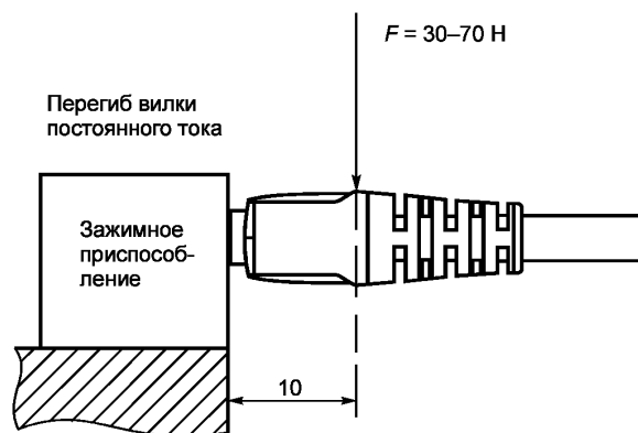
Рисунок С.3 — Прочность на перегиб
