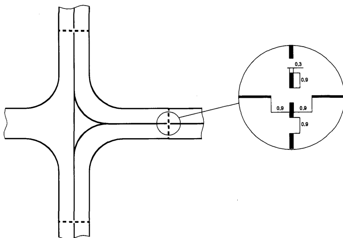
Рисунок 6. Схема маркировки промежуточного места ожидания у пересечения РД
