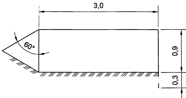
Рисунок 6. Маркер зоны приземления
