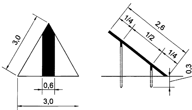
Осовой маркер между концом ЛП и БПРМ
