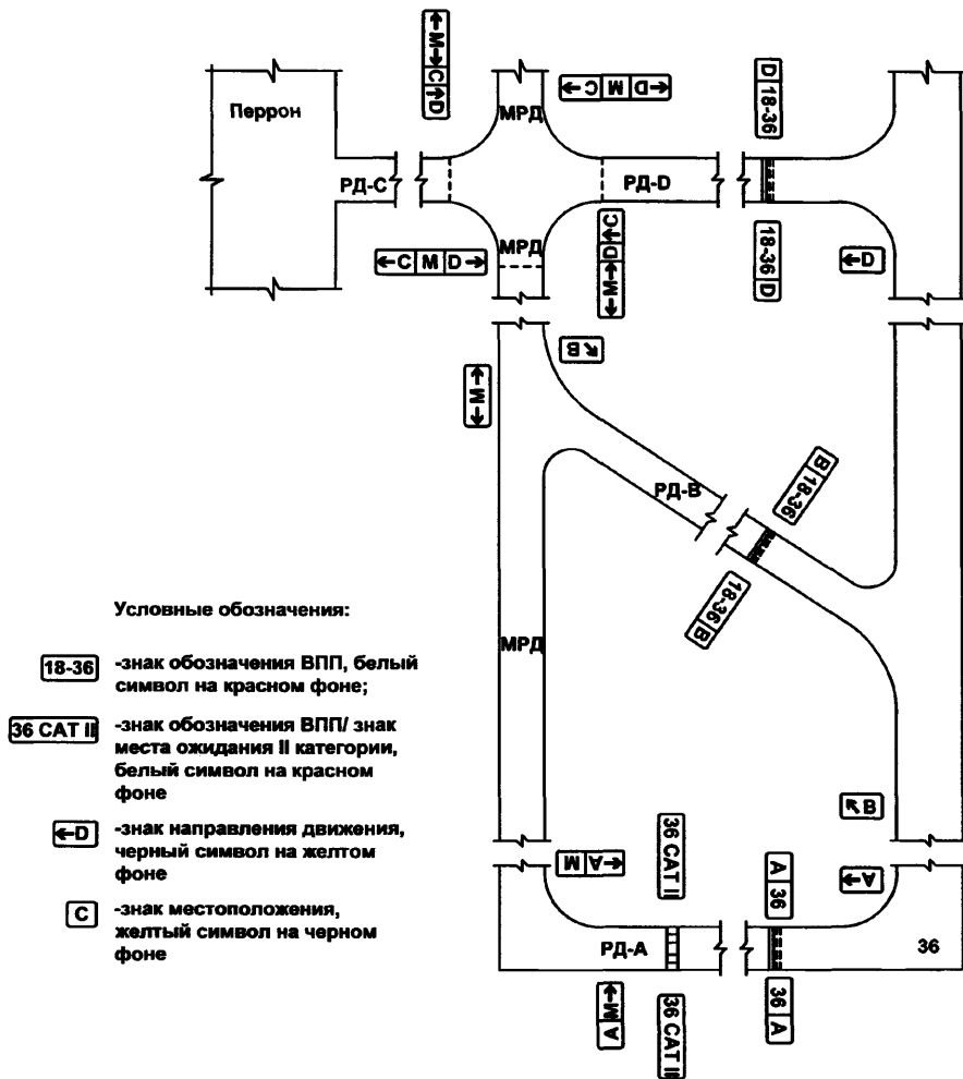
Рисунок 4. Пример расположения аэродромных знаков
