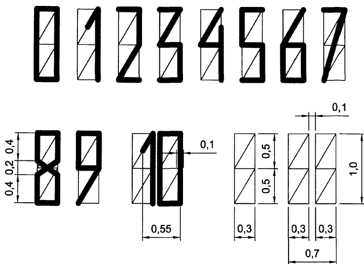
Рисунок 9. Размеры и форма цифр на МС и перроне
