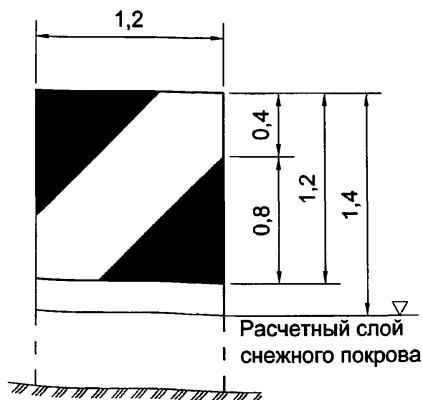
Рисунок 8. Маркер боковой границы
