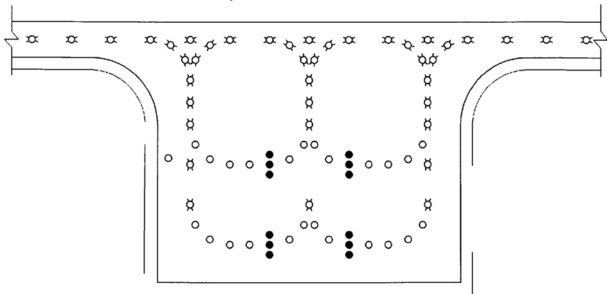
Рисунок 18. Огни защиты ВПП
