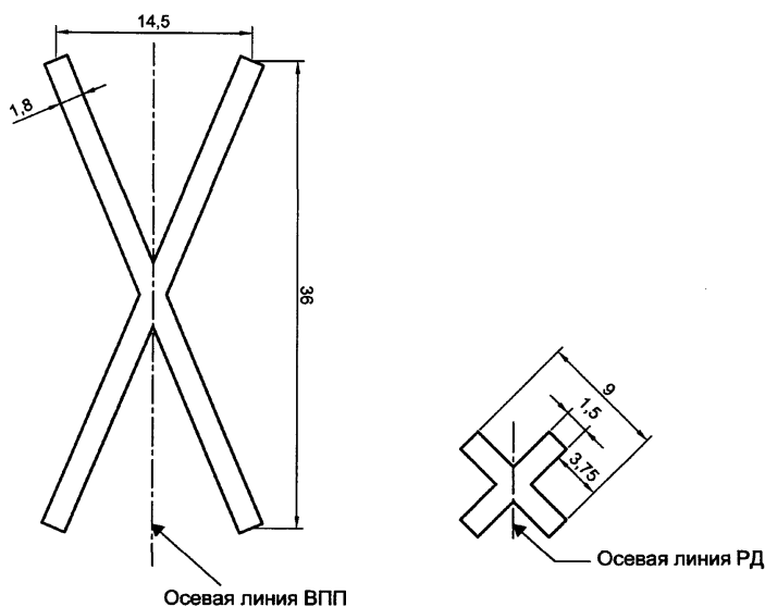
Рисунок 10. Маркировка закрытых для движения ВПП и РД
