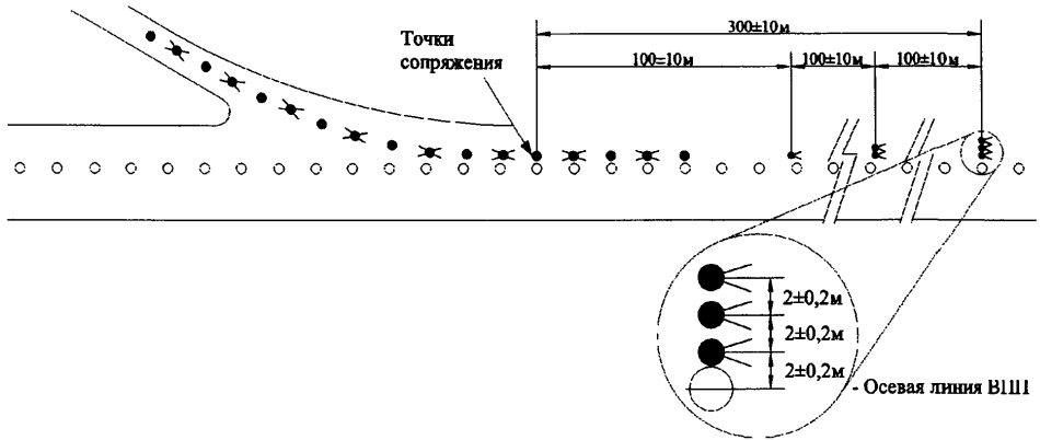
Рисунок 13. Огни указателя РД быстрого схода с ВПП.
