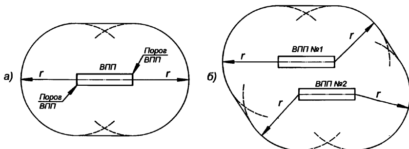
Рисунок 3. Внутренняя горизонтальная поверхность
