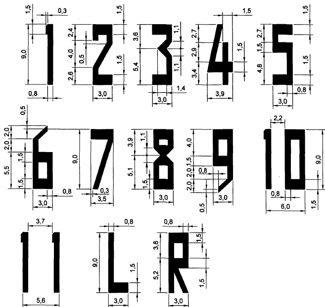
Рисунок 4. Размеры и форма цифр и букв на ИВПШ
