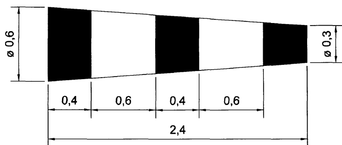
Рисунок. Конус-ветроуказатель
