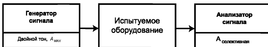
Рисунок 17 — Интермодуляционный метод
