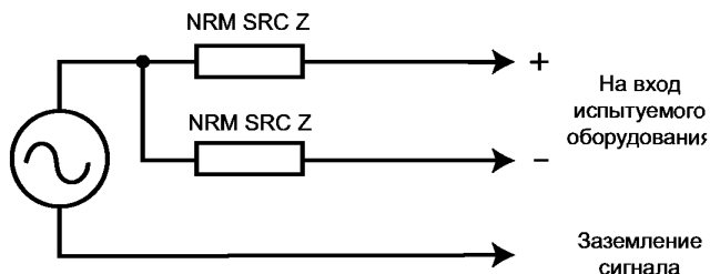
Рисунок 34 — Метод измерения коэффициента подавления синфазного сигнала
