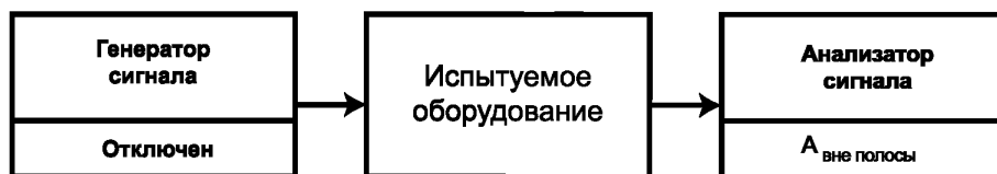
Рисунок 25 — Метод измерения отношения шумов вне полосы
