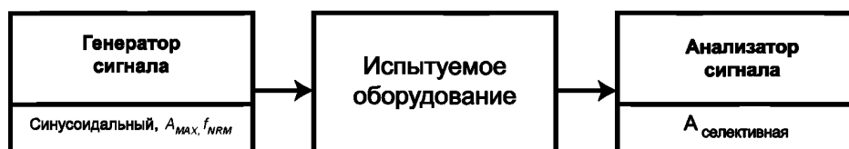
Рисунок 14 — Метод измерения искажения индивидуальных гармоник
