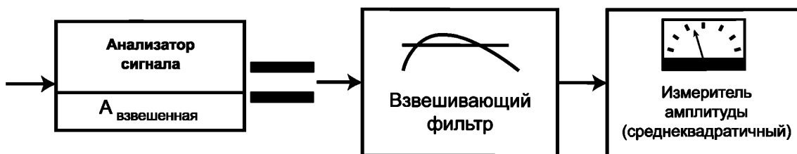
Рисунок 7 — Взвешенная амплитуда
