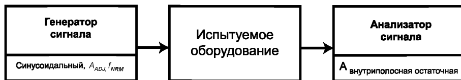
Рисунок 33 — Метод определения функционирования при перегрузке
